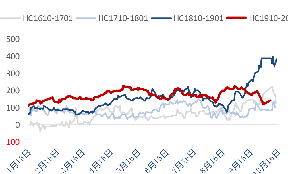
图14：热卷10-1价差
